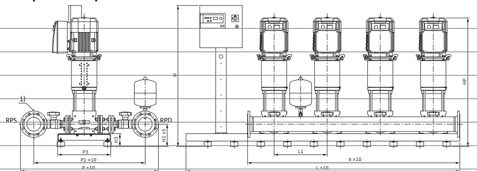
Габаритный чертеж
